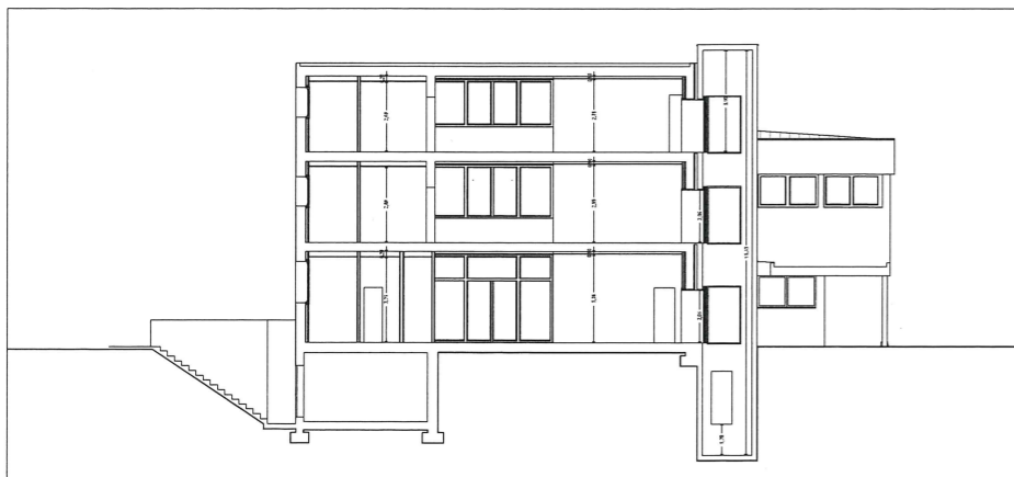
SEZIONE A-A 1:100
